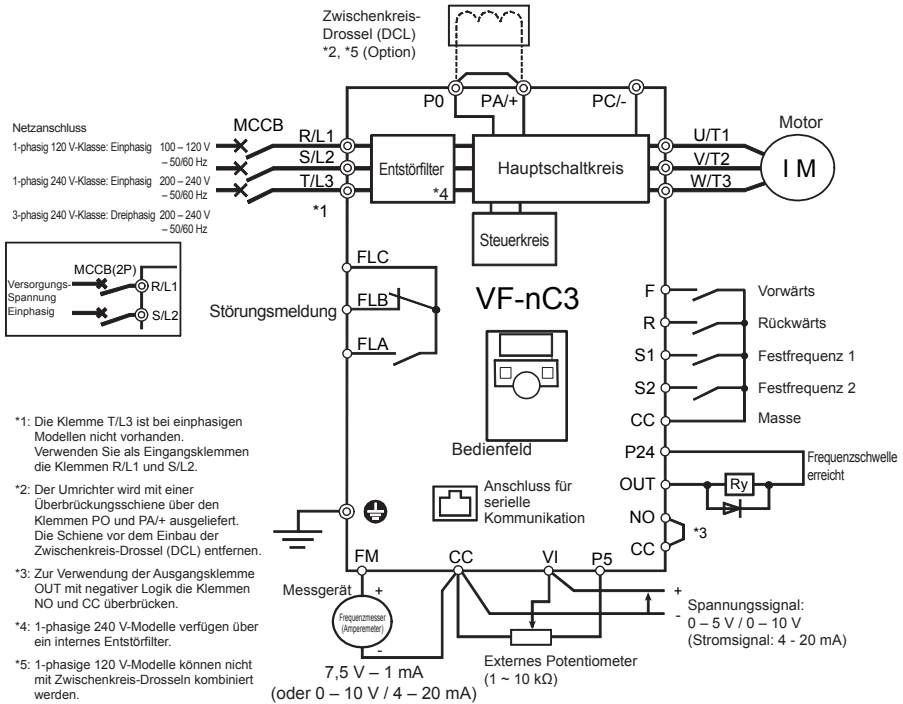
Anschlussdiagramm – negative Logik (SINK) (gemeinsam: CC)
