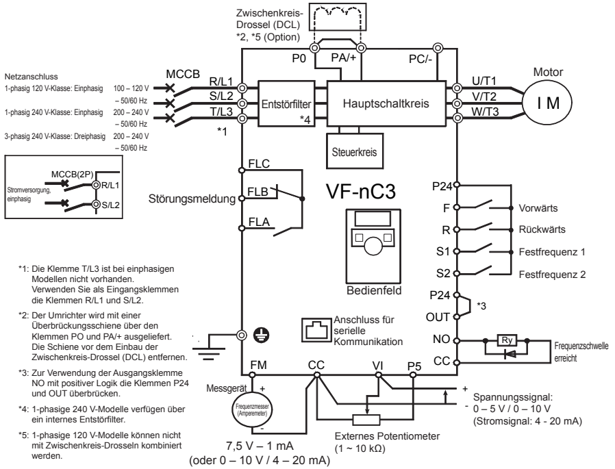
Anschlussdiagramm – positive Logik (SOURCE) (gemeinsam: P24)
